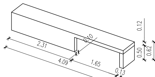
BANCO | Esc.: 1:50 |
