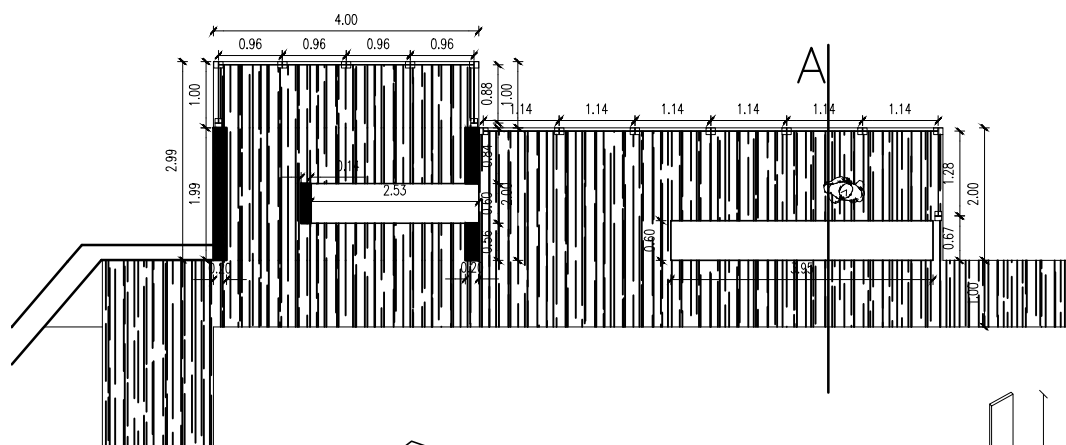
PLANTA | Esc.: 1:75 |
