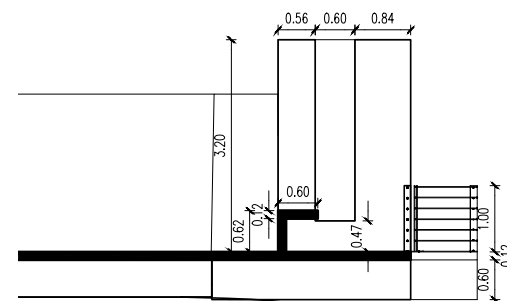
CORTE A | Esc.: 1:75 |
