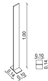
POSTE DE BARANDA | Esc.: 1:20 |
